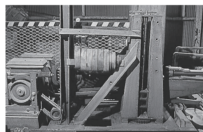
重錘型緊張機（技術研究所に保管）
