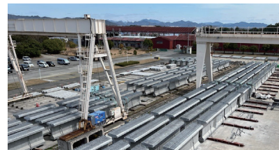
平野東高架橋
