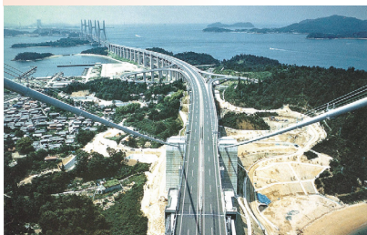
本州四国連絡橋児島坂出ルート・榎島高架橋(香川県) 当社をスポンサーとする国内初のPC専門企業JVでの施工。道路上下線と鉄道を1台で施工でき、道路幅の変化に応じて横移動も可能な大型移動支保工(サポートタイプ)を開発
