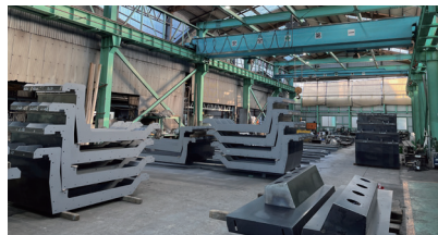
橋桁用鋼製型枠製作状況
