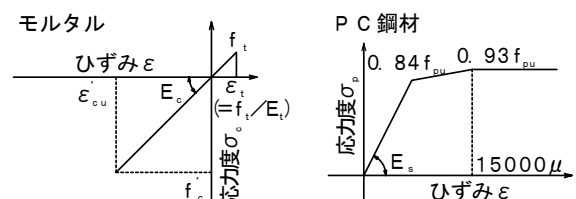
図-4 材料の非線形特性
