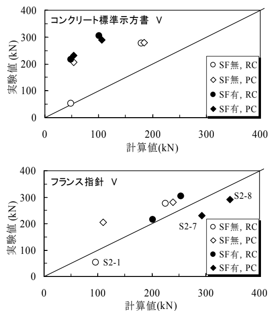
図－10 セン断耐力の実験値と計算値との比較
