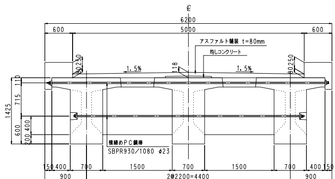
図 - 1 当初設計断面図
