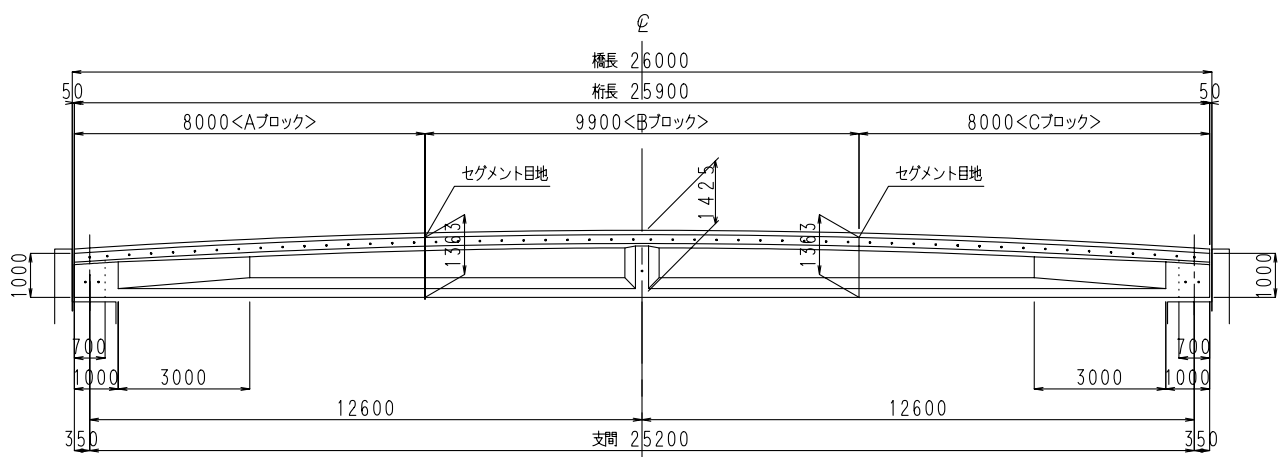
図 - 2 当初設計側面図
