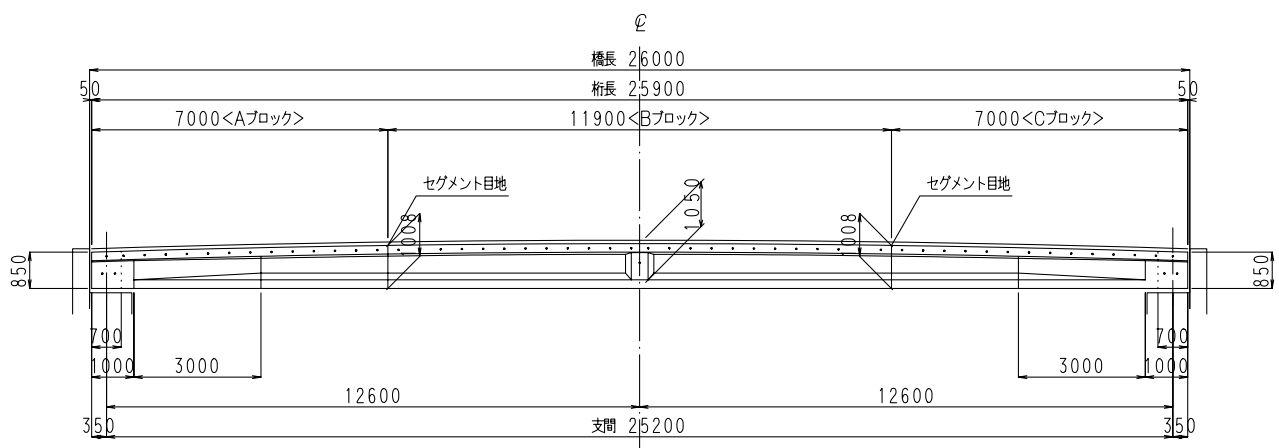
図 - 6 ダックスビーム工法側面図
