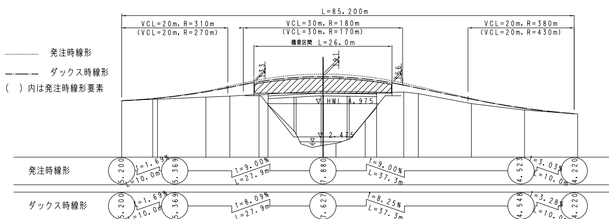
図 - 3 縦断線形要素
