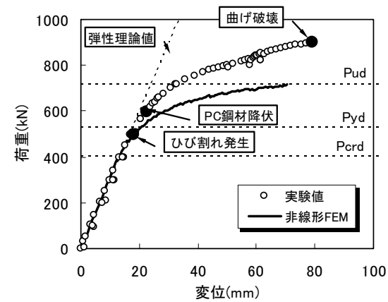
図－３ 荷重－変位曲線の結果
