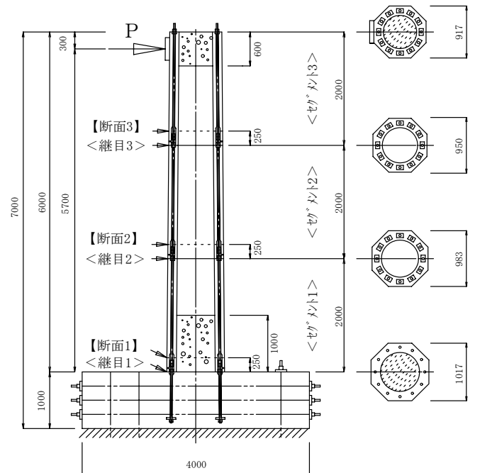
図－２ 供試体一般図
