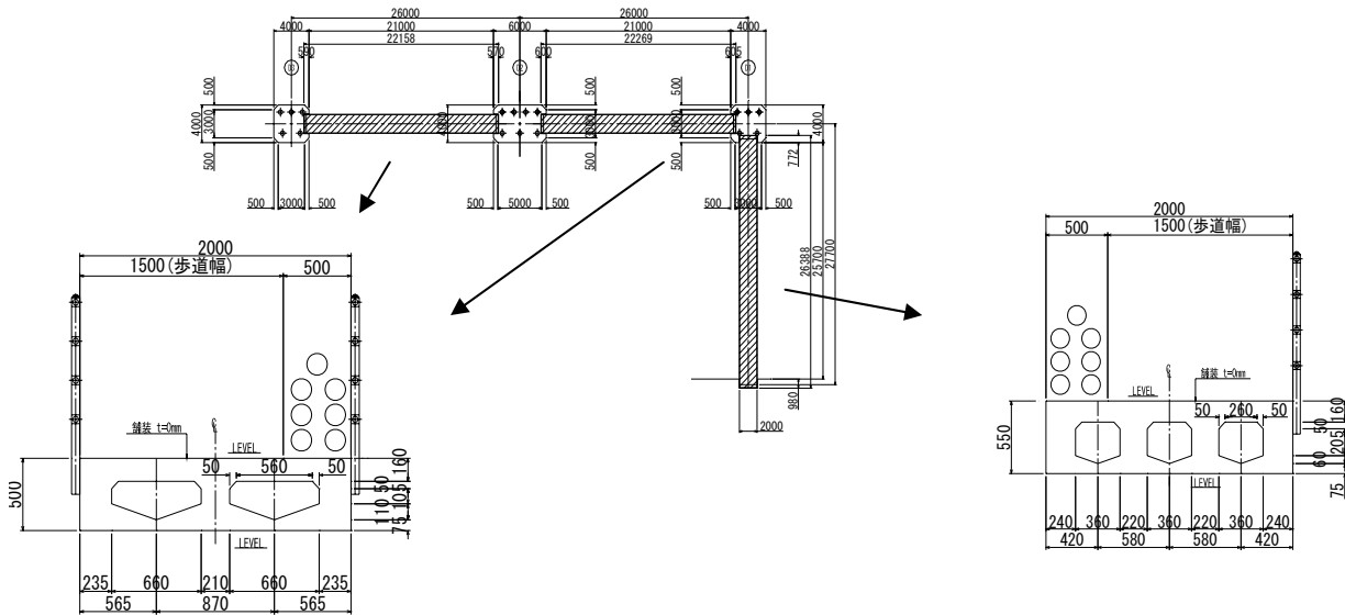
図-1 平面形状及び断面図
