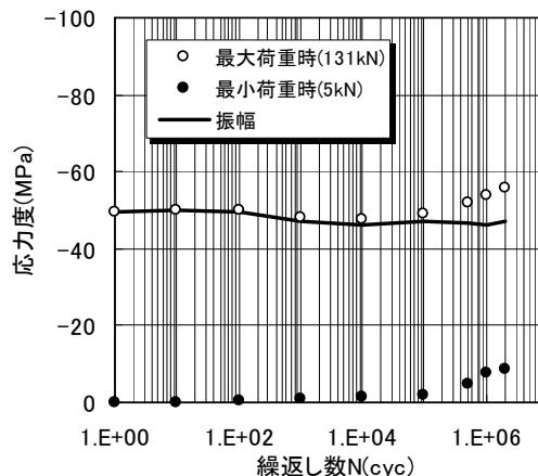
図-5 繰返し数と桁上縁応力度との関係
