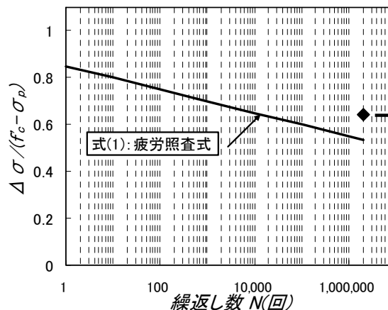
図-6 変動応力比と繰返し回数との関係
