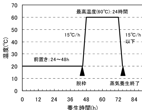
図-2 養生方法
