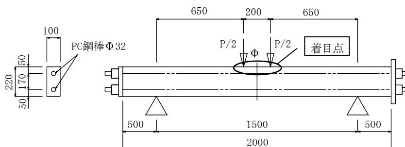
図-1 供試体一般図
