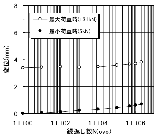
図-4 繰返し数と変位との関係
