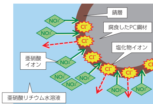
水溶液注入直後
