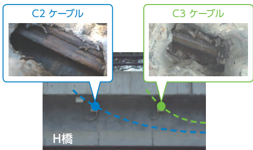
施工前のPC鋼材の腐食状況とモニタリング位置
