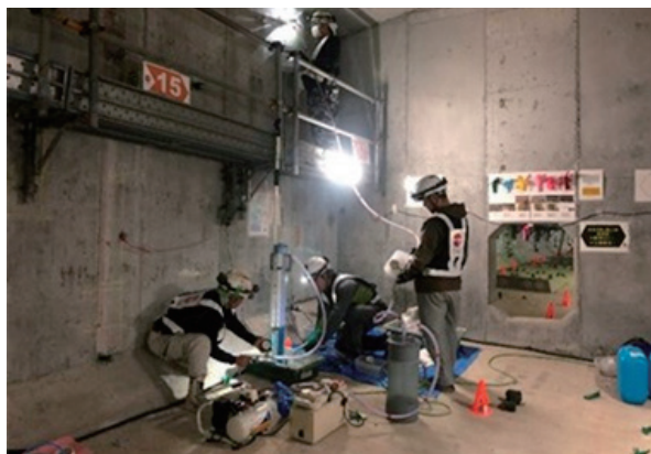
水溶液・補修材充填
