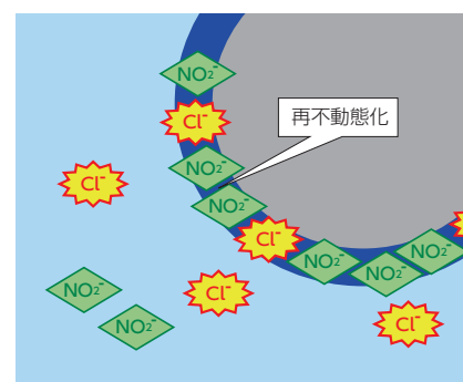
PC鋼材表面の再不動態化
