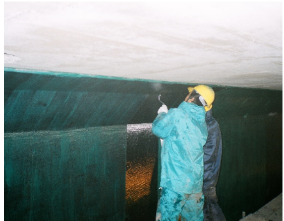
【炭素繊維プレート 主桁曲げ補強】
