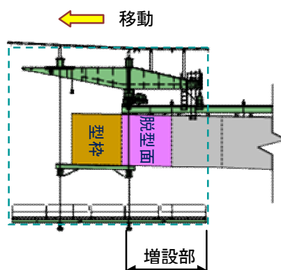
図-7 移動式作業車後方の増設
