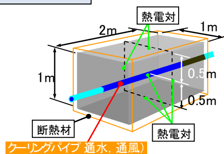
図-3 マスコンクリート供試体
