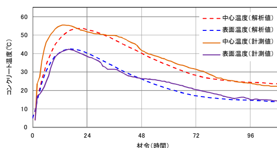
図-6 コンクリートの温度履歴（2リフト）
