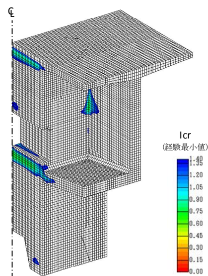
図-5 ひび割れ指数(Icr)分布
