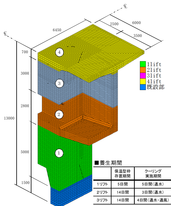
図-4 解析により決定した養生条件
