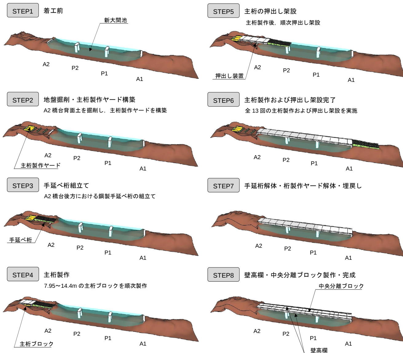
図-3 施工ステップ図
