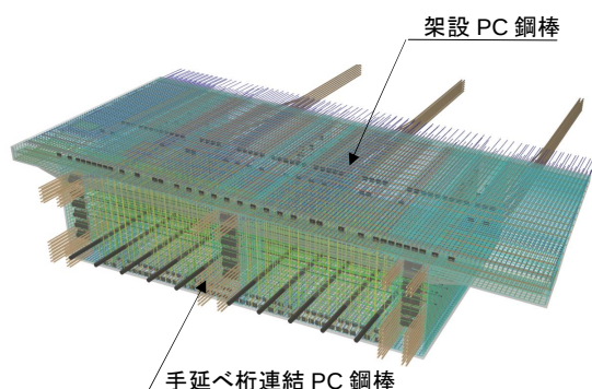
図-4 CIM モデル(A1 端部ブロック)
