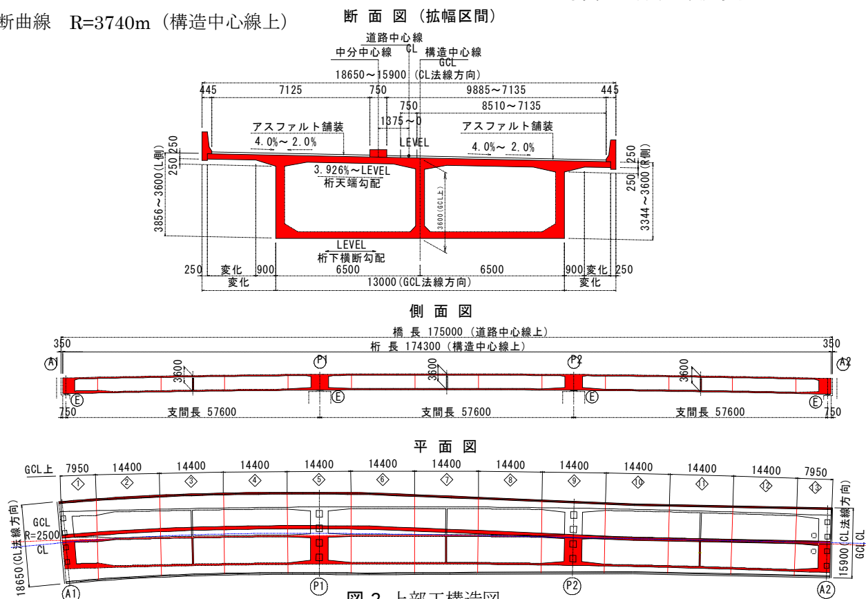
图-2 上部工構造図
