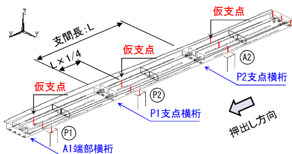
図-3 FEM 解析モデル(仮支点が支間 1/4 位置)
