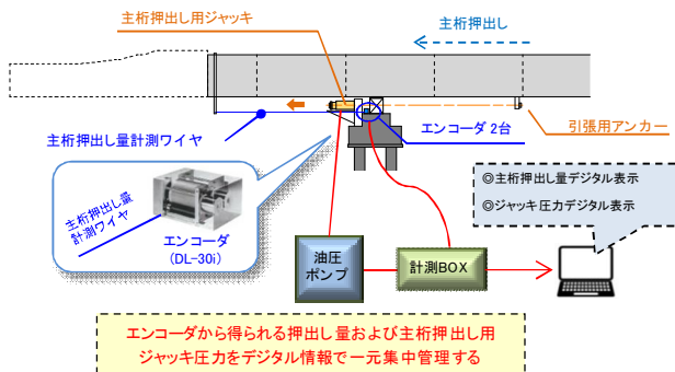
図-7 一元集中管理概要図
