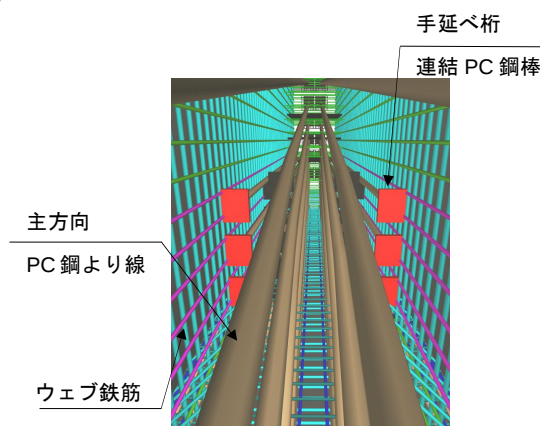
図-5 CIM モデル(ウェブ内の干渉チェック例)
