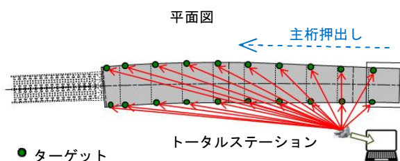
写真-5 トータルステーション計測
