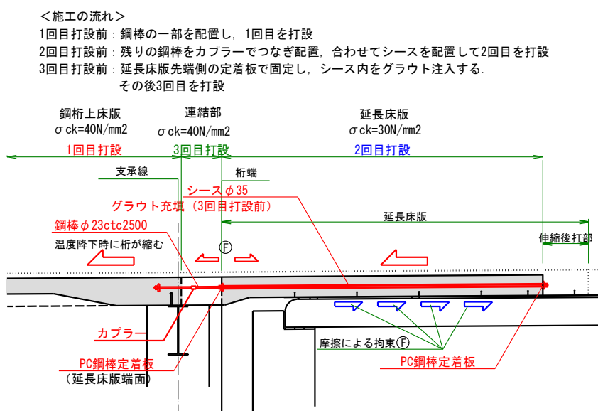
図-6 PC 鋼棒による固定方法概要図
