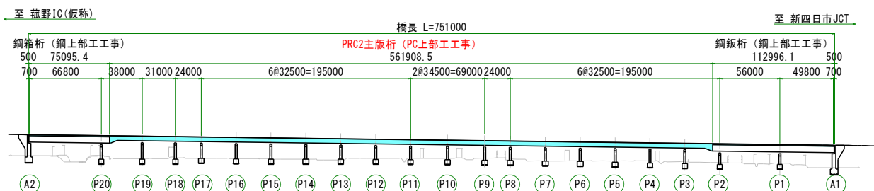
図-3 構造一般図 (上り側面図)
