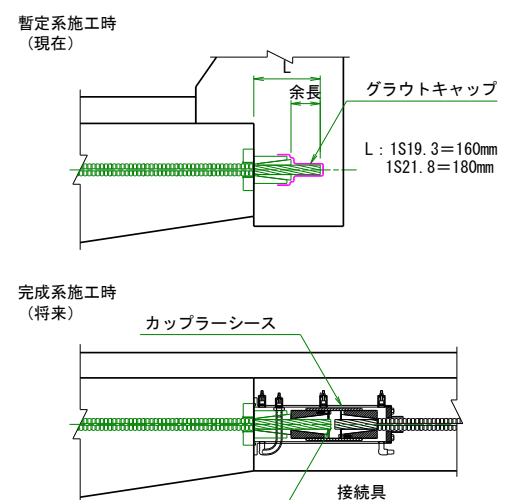
図-9 将来拡幅のための床版横締め処理概要図
