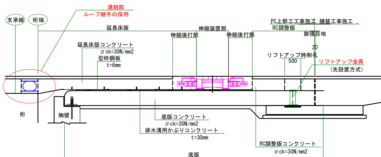
図-5 延長床版構造概要図
