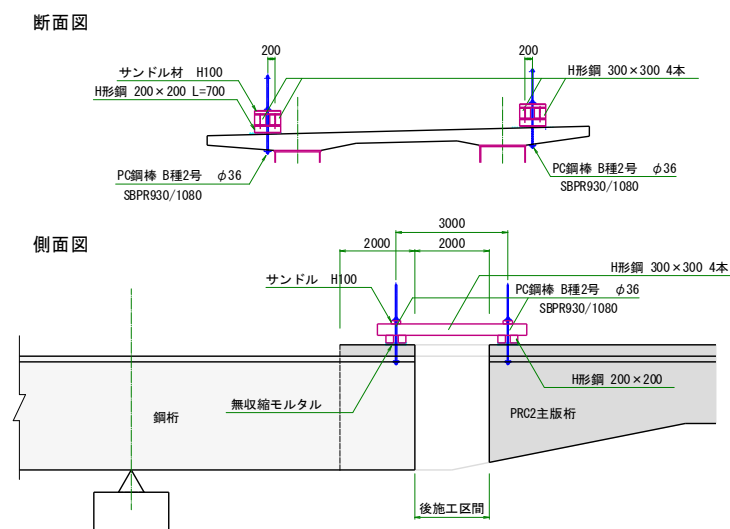
図-4 変位拘束鋼材概要図
