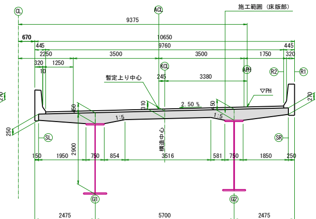
図-2 構造一般図 (上り断面図)
