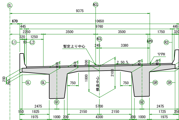
鋼箱桁部
