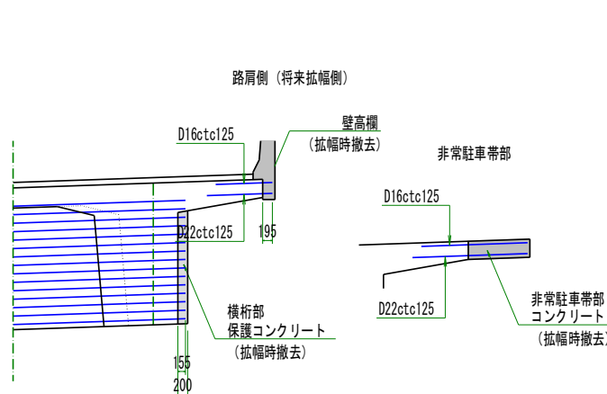
図-8 拡幅用鉄筋の配置概要図
