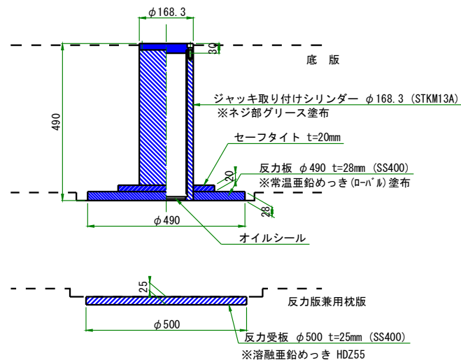
図-7 リフトアップ金具図
